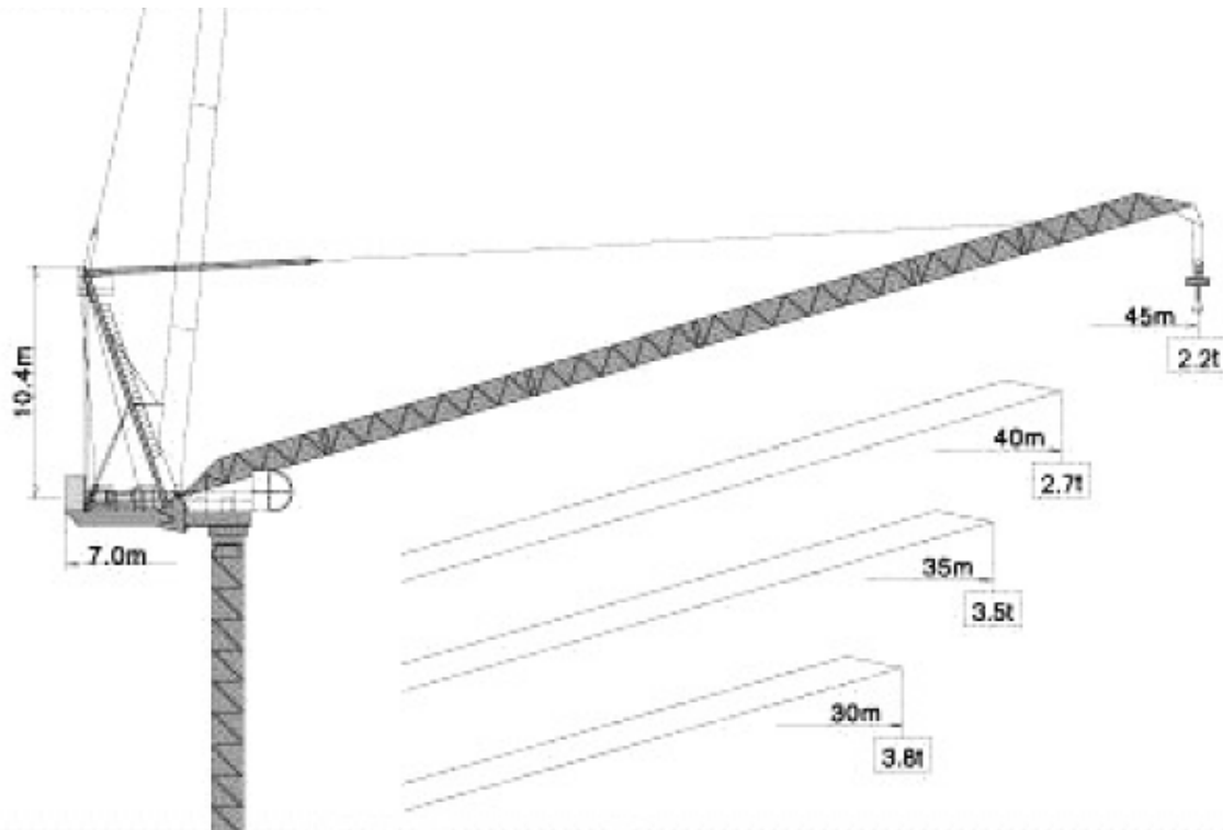
塔身截面 Mast:2m x 2m
