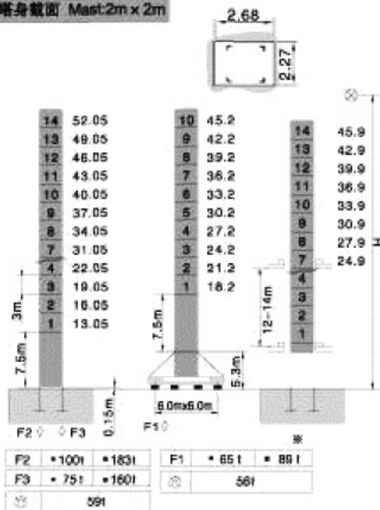
塔身截面 Mast:2m x 2m
