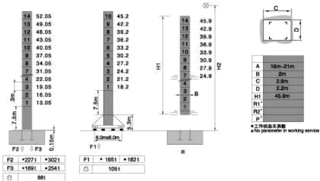
塔身截面 Mast: 2m x 2m
