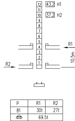
内爬式 Internal climbing
