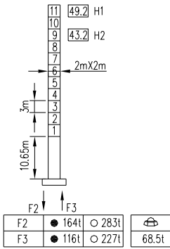
固定式 Stationary
