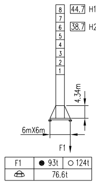
行走式 Travelling
